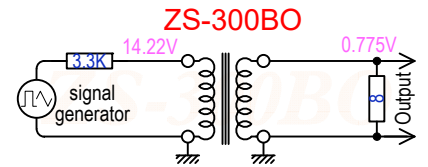
Fig 1. 静态测试(Static Test)
